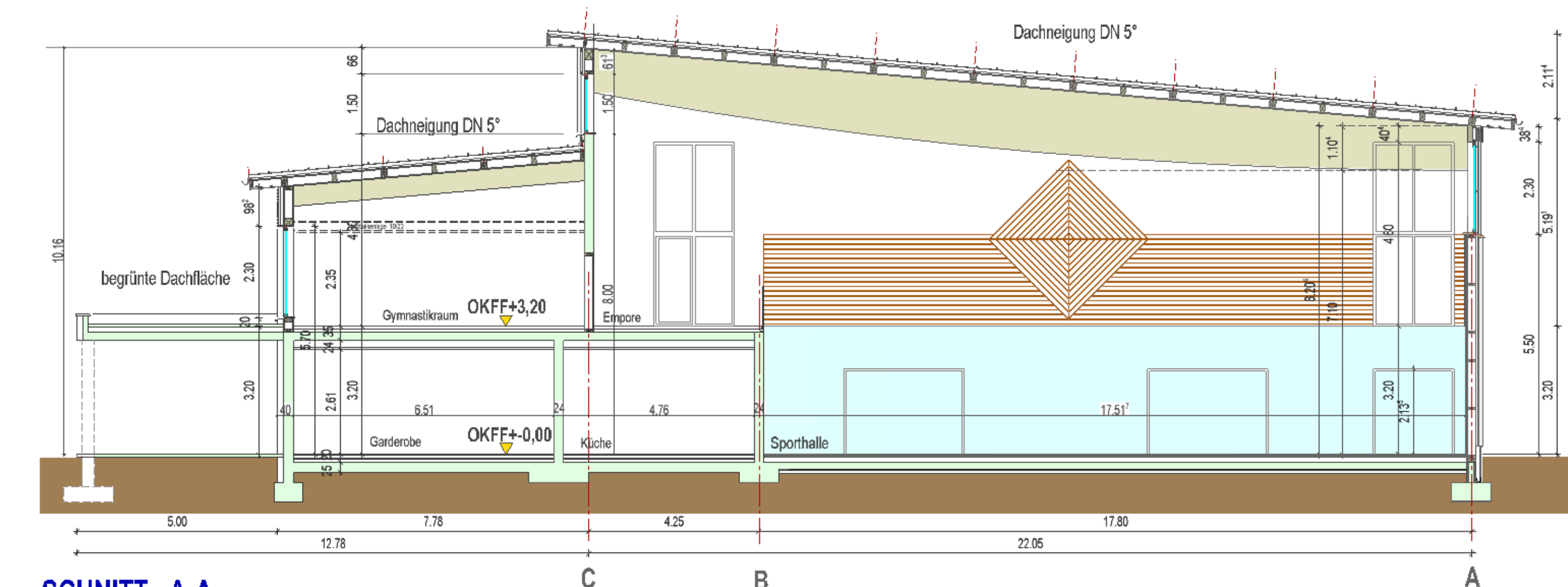
SCHNITT A-A
